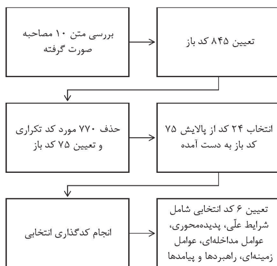
شکل ۱. فرایند کدگذاری
